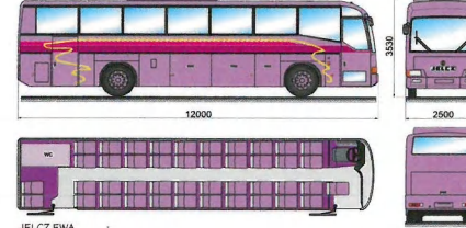
JELCZ EWA
