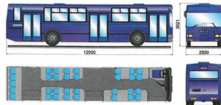
JELCZ 120M, 120MM/1
