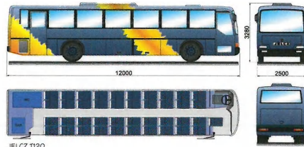
JELCZ T120M
